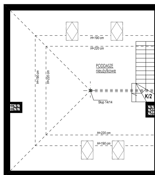
Poddasze nieużytkowe
