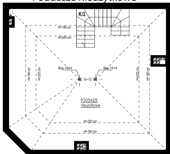
Poddasze nieużytkowe
